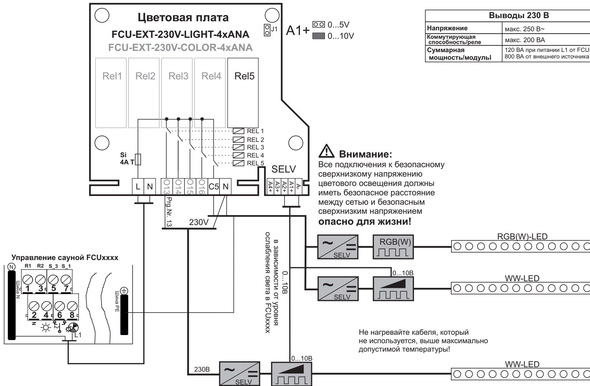
Схема соединений платы цветowego светильника FCU-EXT-230V-Light-4xAна FCU-EXT-230V-Color-4xAна
